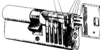
Fúrás elleni védelem fúrásvédő csappal
